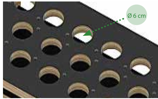
Draufsicht Pinselwagen
